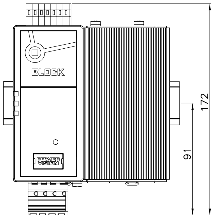
Darstellung mit Anschlußklemmen
