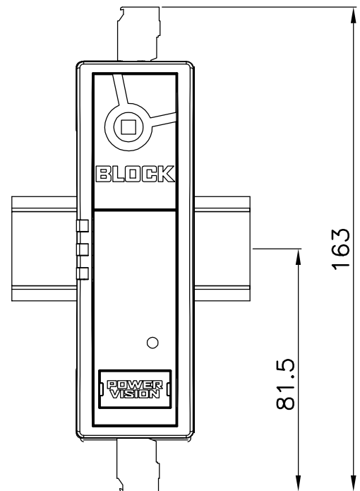
Darstellung mit Anschlußklemmen
