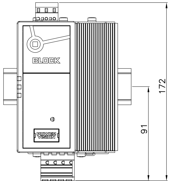
Darstellung mit Anschlußklemmen
