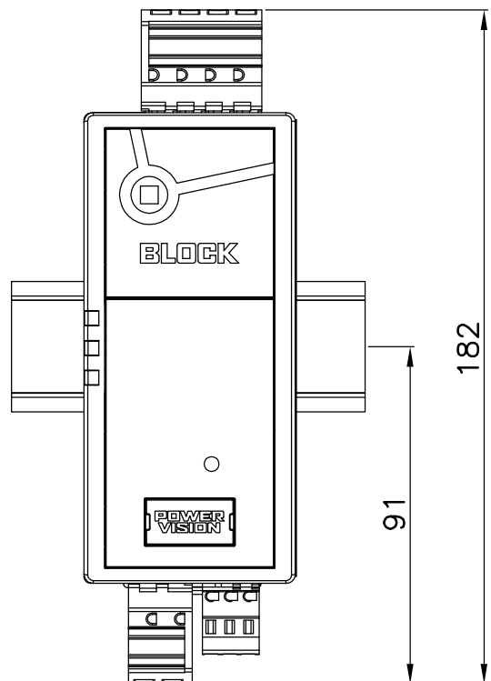
Darstellung mit Anschlußklemmen
